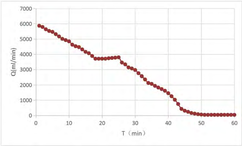
图 7.3.1 SK01渗水试验Q-t曲线图
