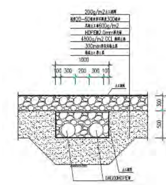
图 9.2-7 主盲沟结构图
