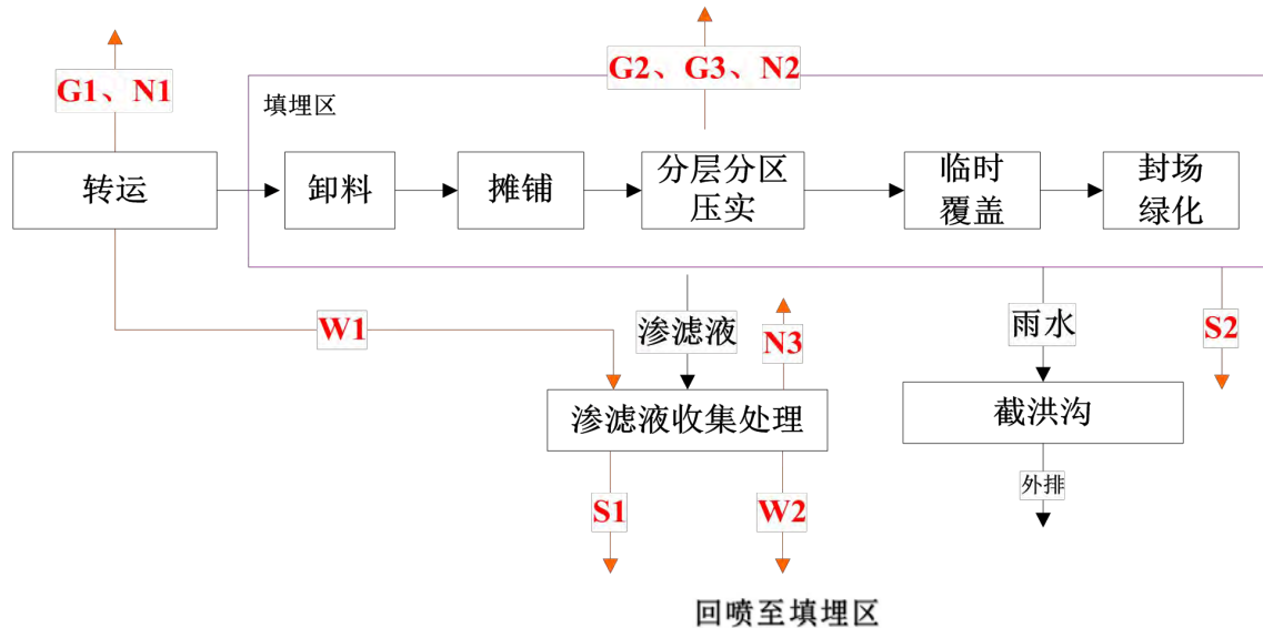
图 4.1-2 本项目工艺流程及产污节点图
