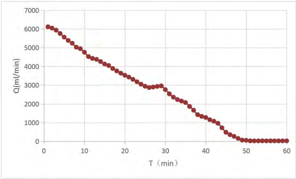
图 7.3-2 SK02渗水试验Q-t曲线图
