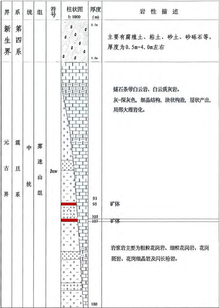
图5.1-7 地层综合柱状图
