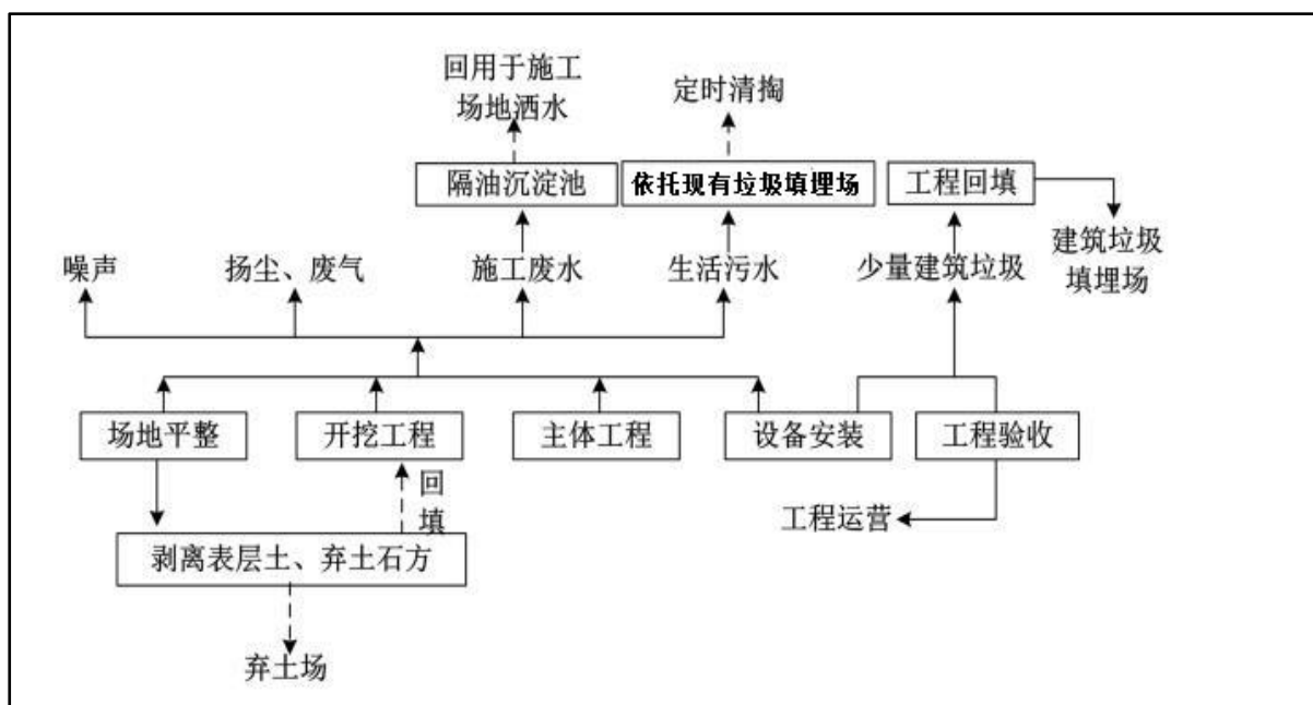
图4.1-1 施工期工艺流程及产污情况图
