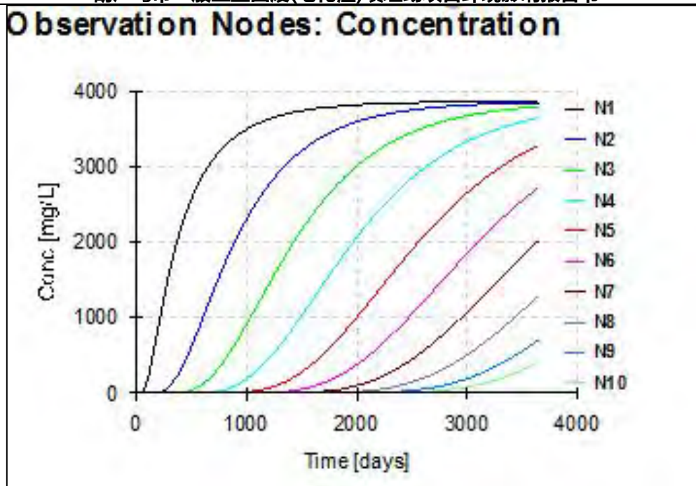
图 7.6-2 氯化物在本次预测各深度浓度变化趋势
