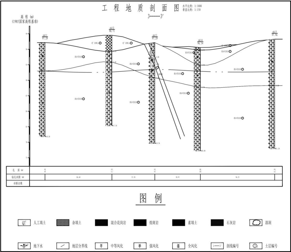
图7.3-6 项目区域地质剖面图3
