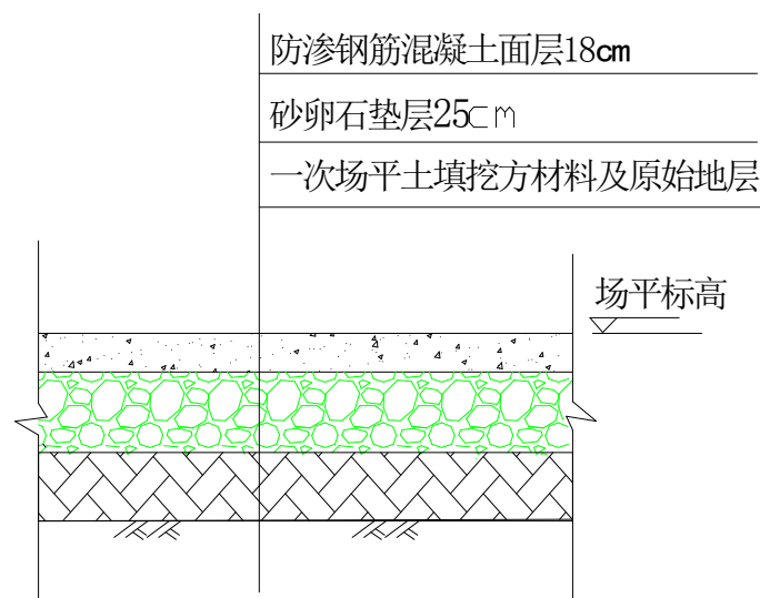
图9.2-2 一般污染防治区典型防渗结构示意图
