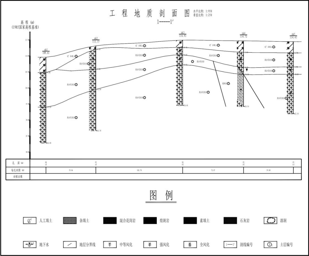
图 7.3-4 项目区域地质剖面图1
