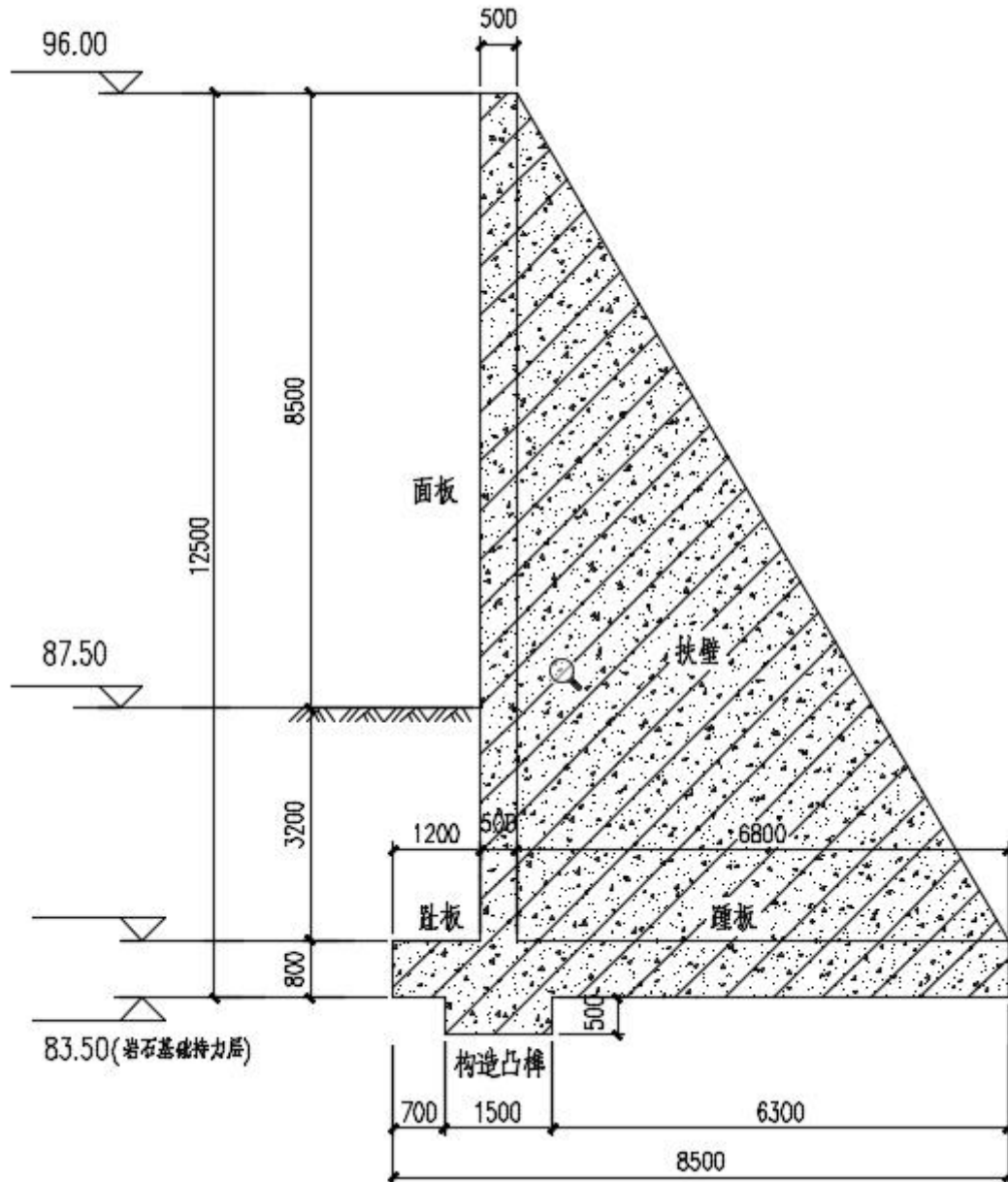
图3.3-6 坝体断面图
