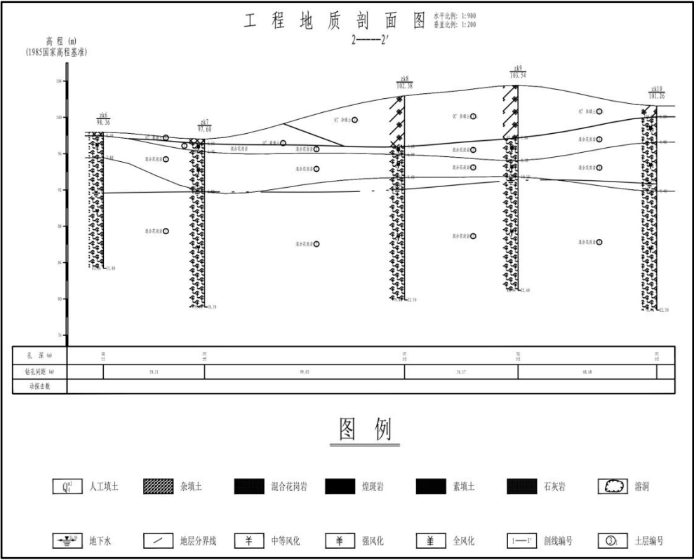
图 7.3-5 项目区域地质剖面图2
