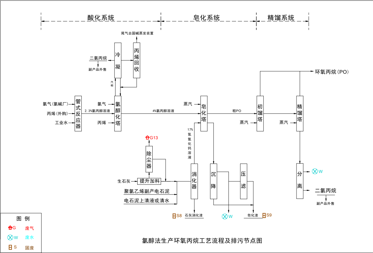
图3.2-1 氯醇法生产环氧丙烷工艺流程及排污节点图
