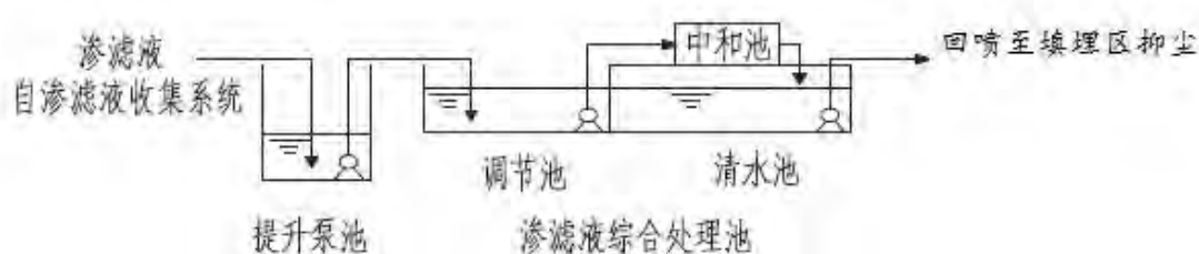
图 3.3-11 本项废水处理工艺流程图
