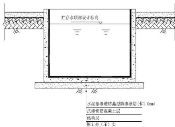
图9.2-4 污水处理池防渗示意图
