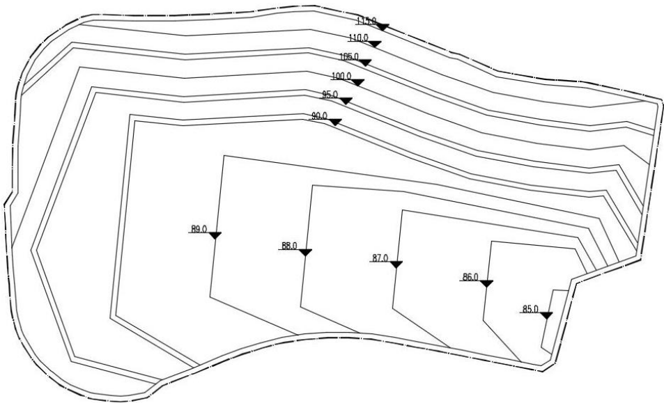
图3.3-4 清场等高线图
