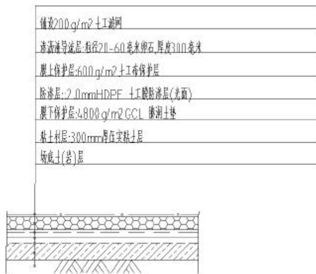
图 3.3-7 底部防渗结构图
