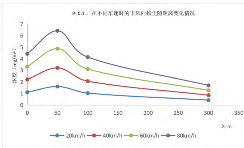
7.1-1 P=0.1 车速为 20km/h -80km/h的下风向扬尘随距离变化情况
