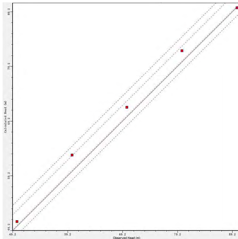
图 7.3-13 区域实测水位与模拟水位拟合
