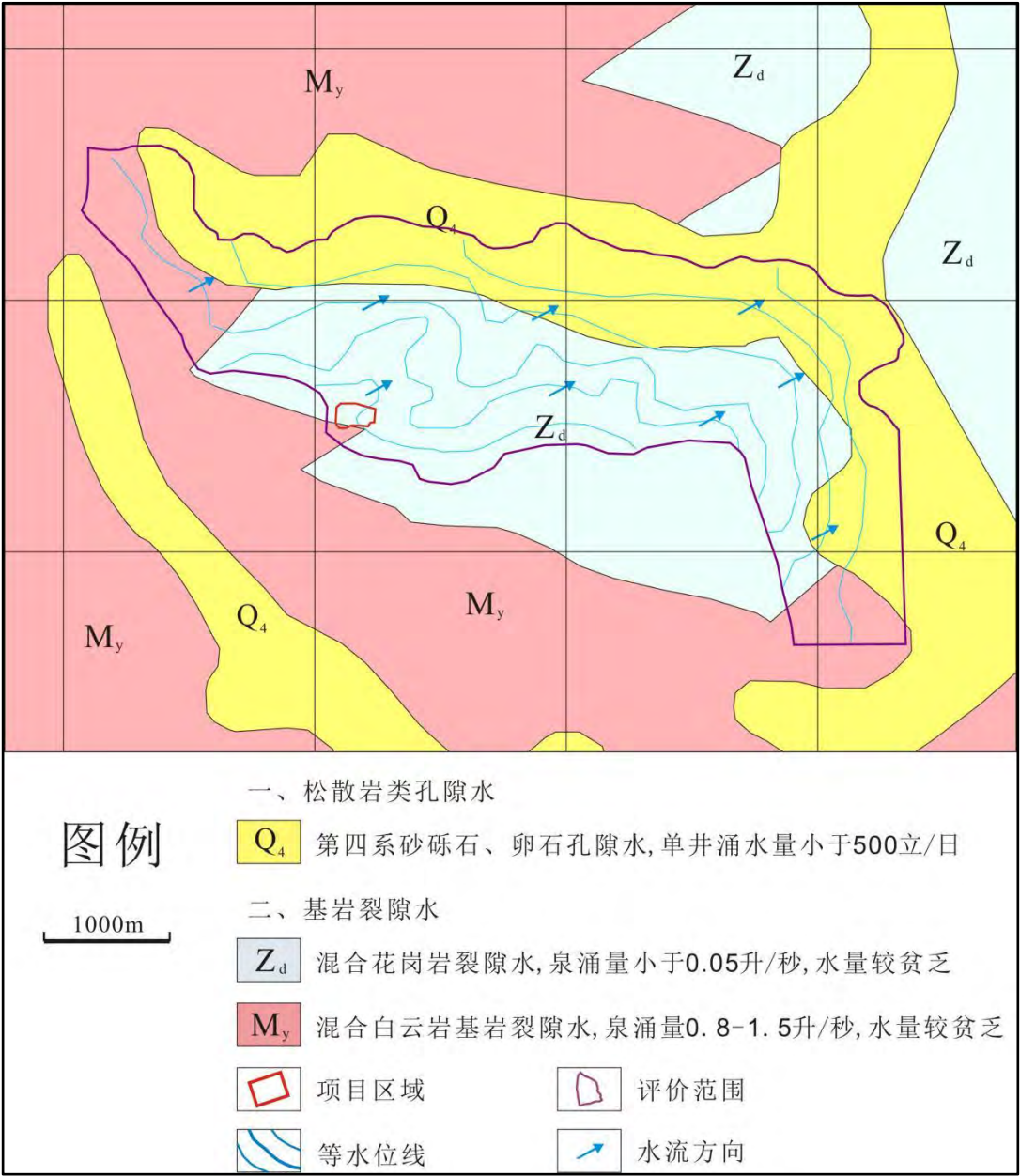
图 7.3-3 区域水文地质图 (1:50000)
