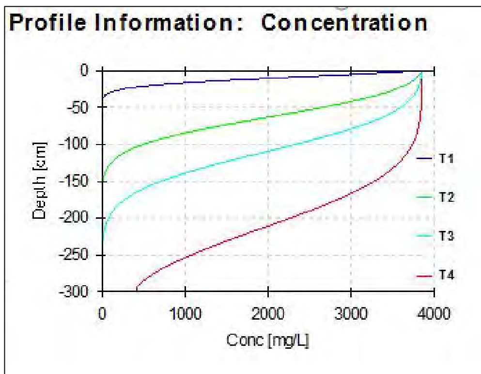
图 7.6-1 氯化物在不同时段的土壤迁移情况
