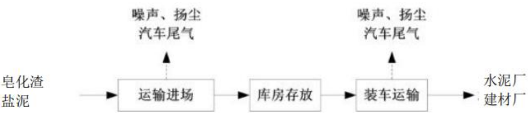
图 3.5-1 工艺流程图及产污节点
